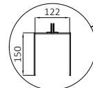
DMR.APR.P1028 Hanging U Apparatus
