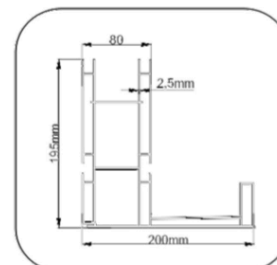
1 - Gronda Travicello
