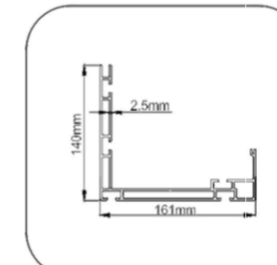
5 - Grondaia Anteriore
