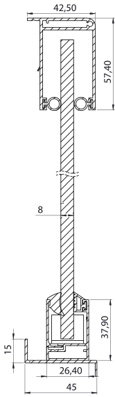
Plus Triangle Vetro Singolo
