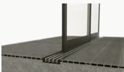
Incassato nel Pavimento con Profilo ad F
