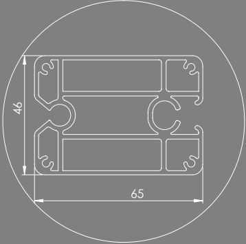
Terminal Profil
